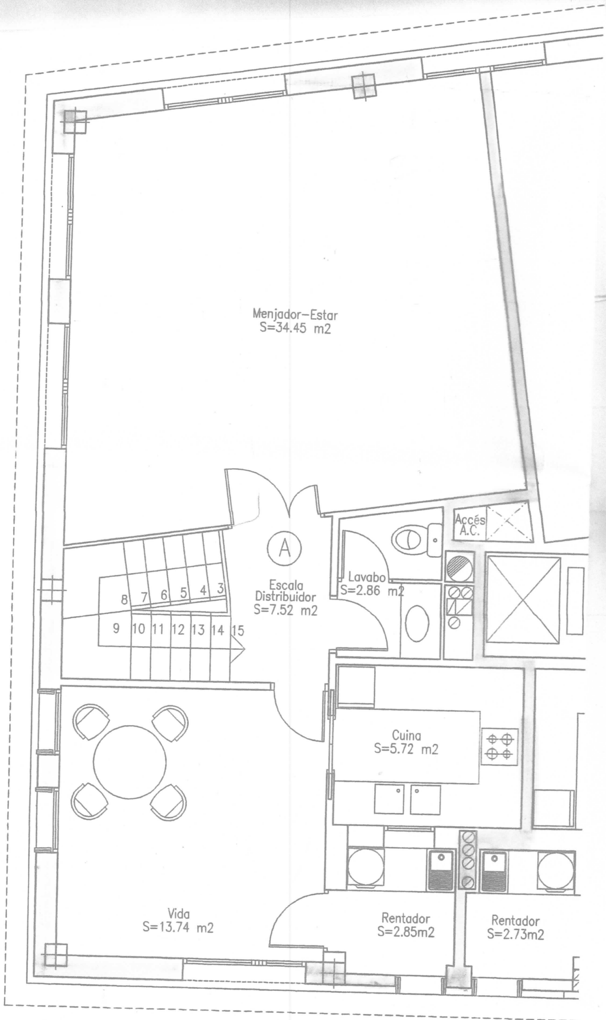
PLANTA SOTACOBERTA
